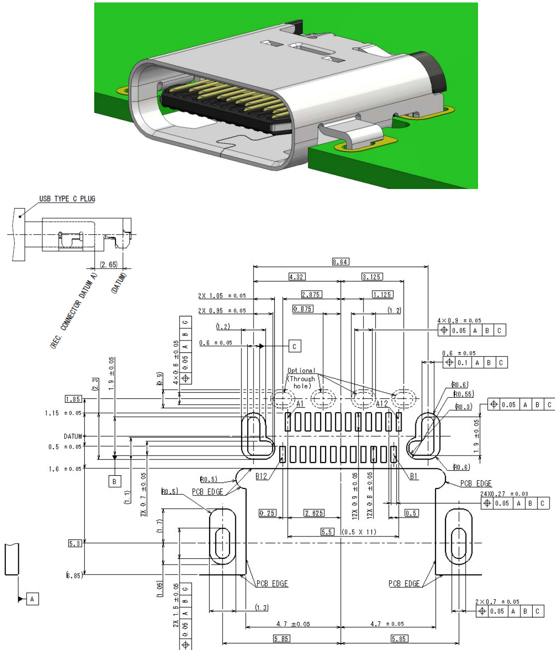
中端双列（沉板）SMT插座
